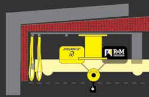
Figura 1. Festón de Pista en C
