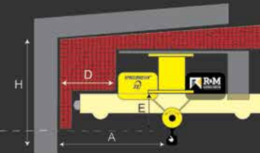
Figura 2. Sistema de Electrificación NRGmaster
